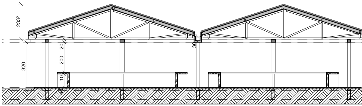
COUPE AA
